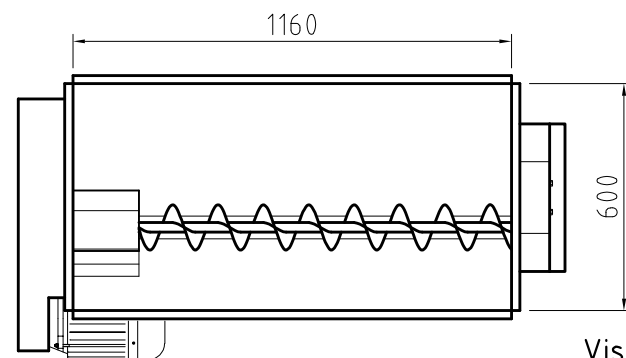
Vista laterale
