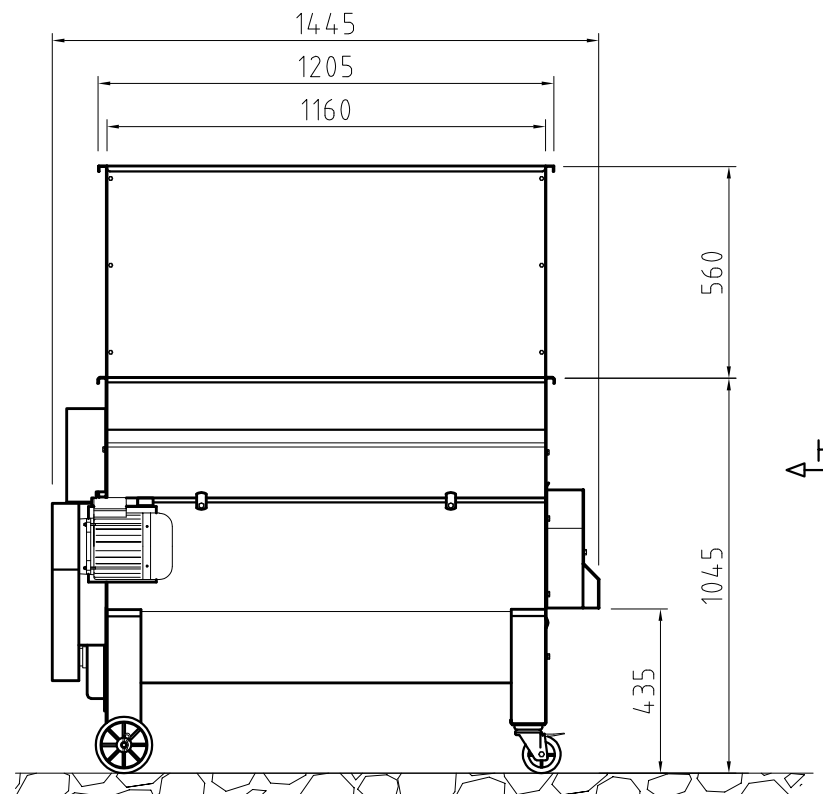
Vista laterale
